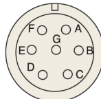
MS3102A20-15P (브레이크 부착형)
