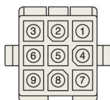
AMP 172161-1 CAP 170362-1 Pin
