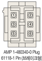
모터 Connector 접속도
